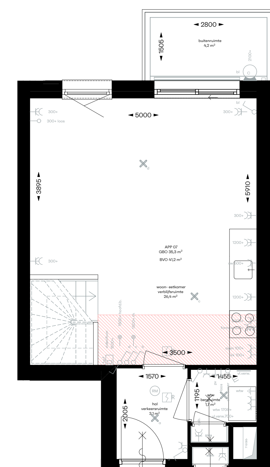
1:50 2e verdieping
