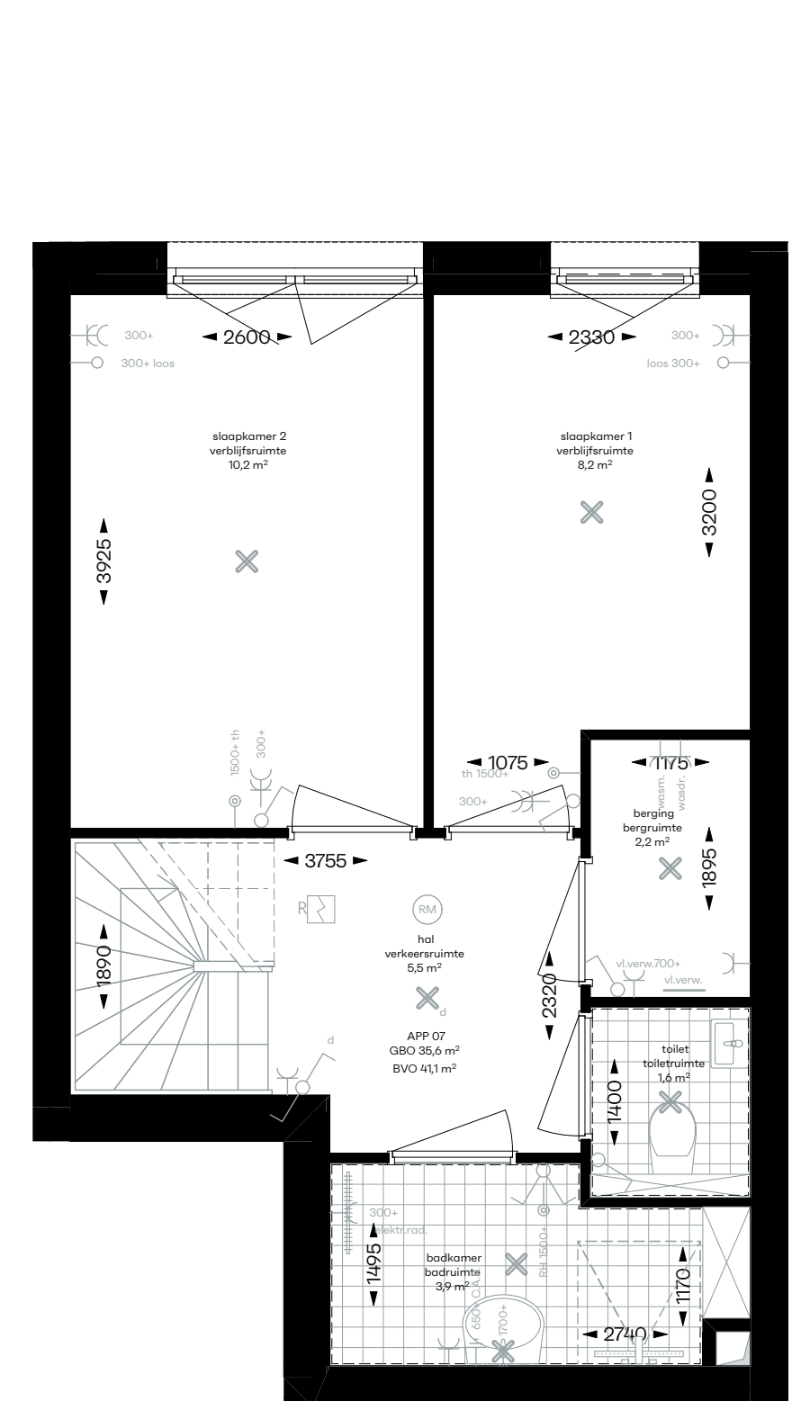
1:50 1e verdieping
